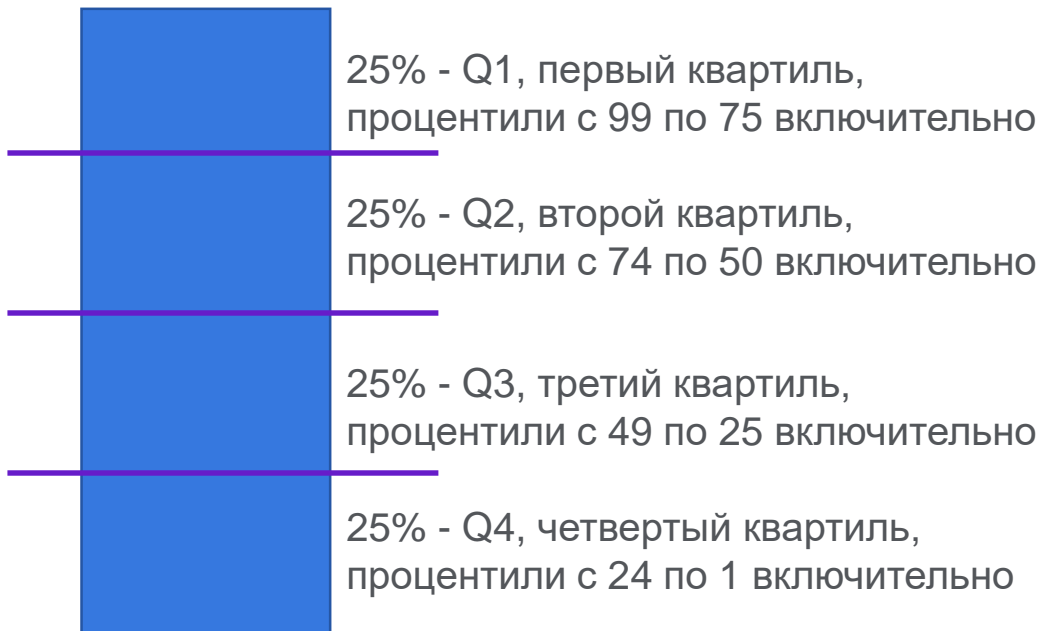
Квартили
